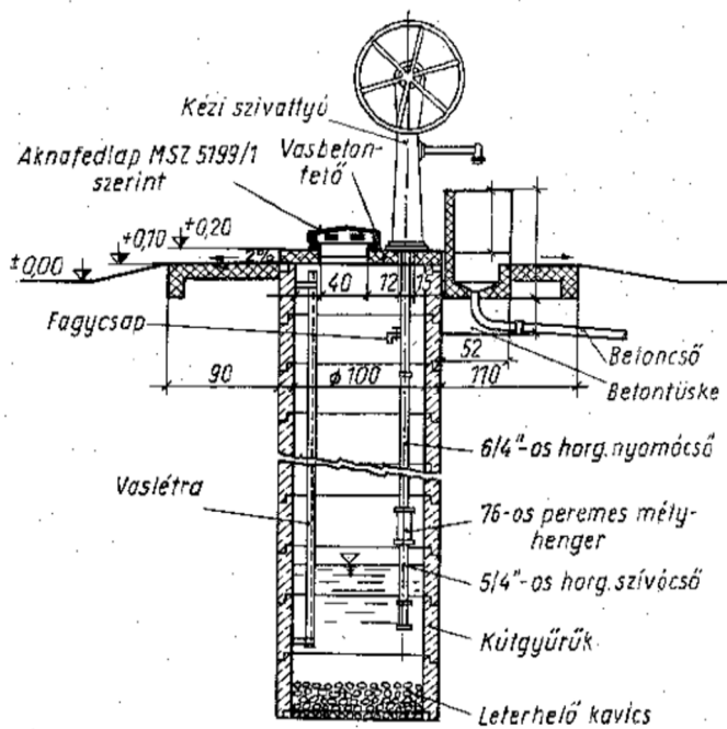
4. ábra. Betongyűrűs ásott kút szabványos kiképzése
